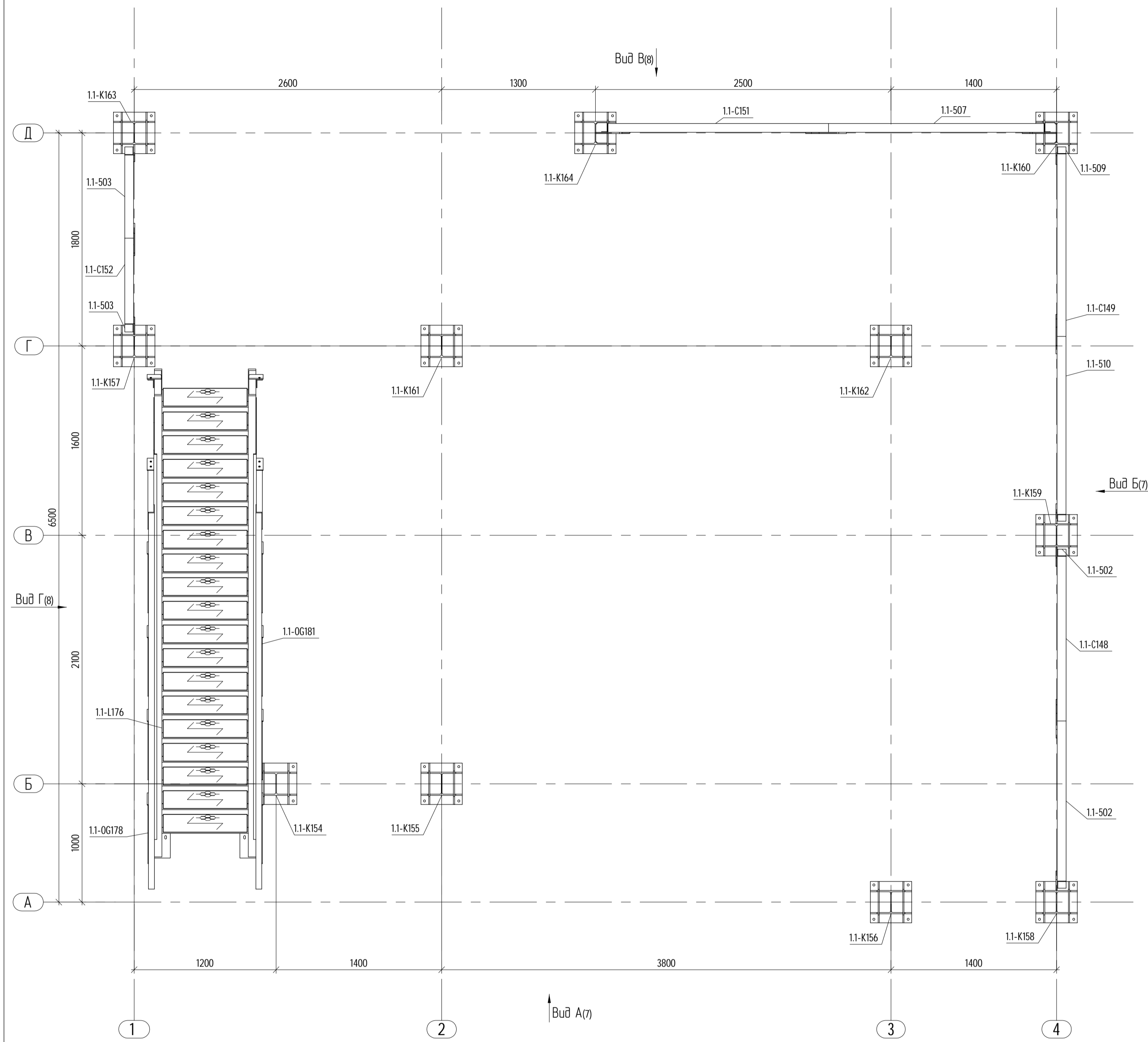
План колонн на отм. 0.000
