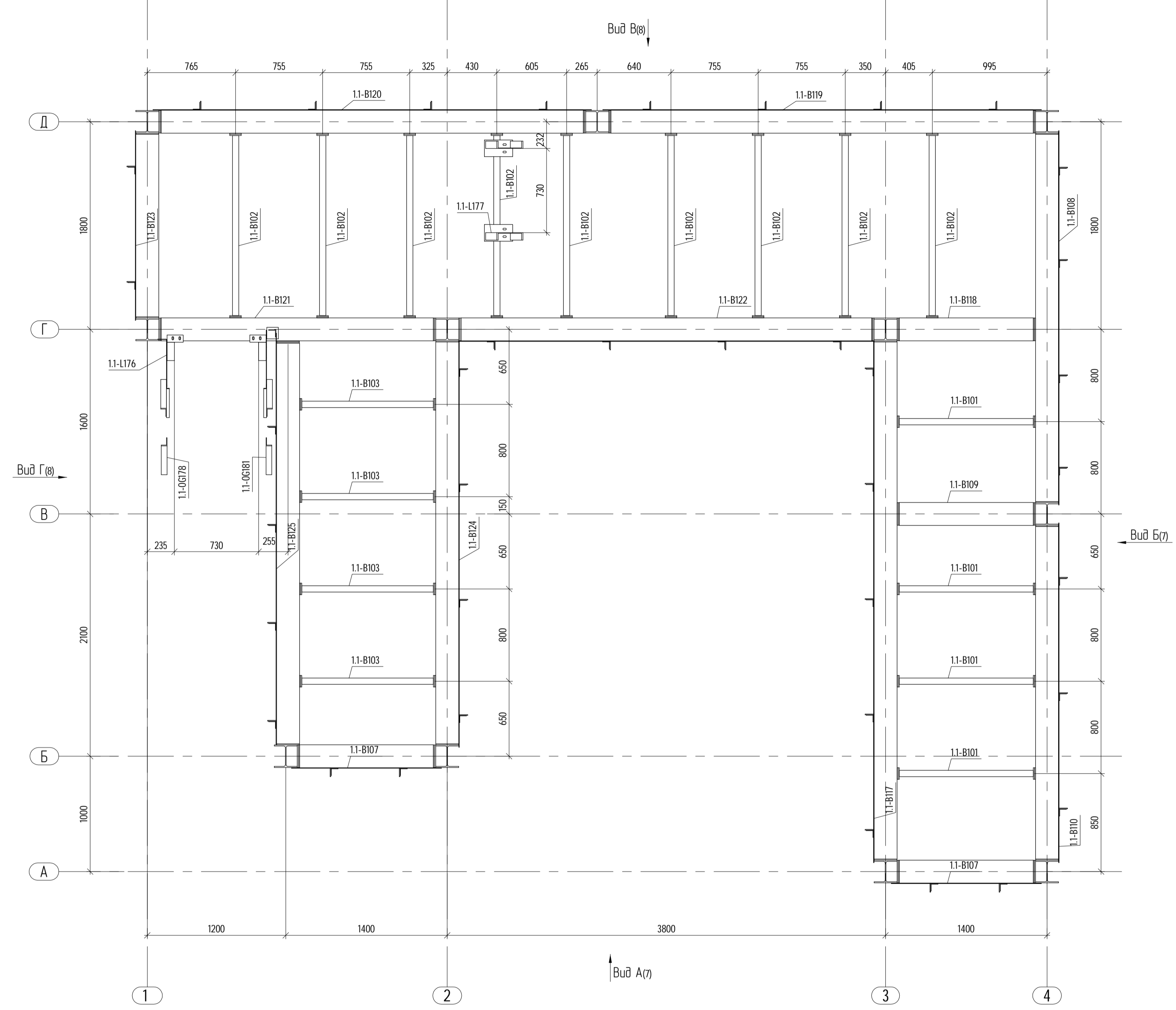
План настилов на отм. 4.200 (настилы условно не показаны)
